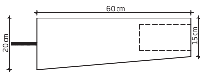
VISTA LATERAL
