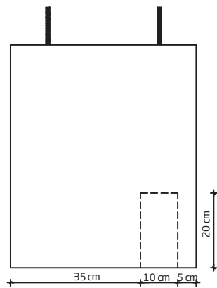
VISTA POSTERIOR
